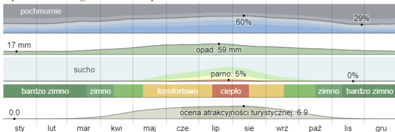
Wykres 3. Klimat w gminie Łaziska na przestrzeni roku
