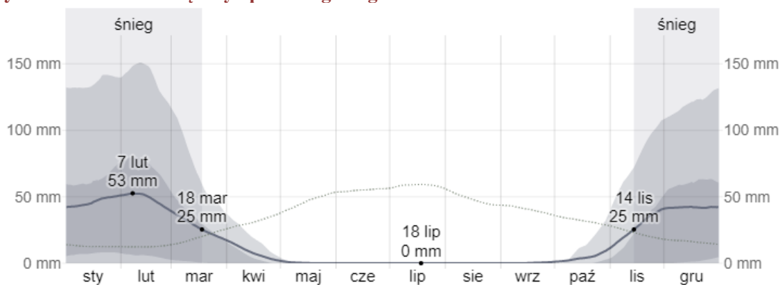
Wykres 5. Średni miesięczny opad śniegu w gminie Łaziska
