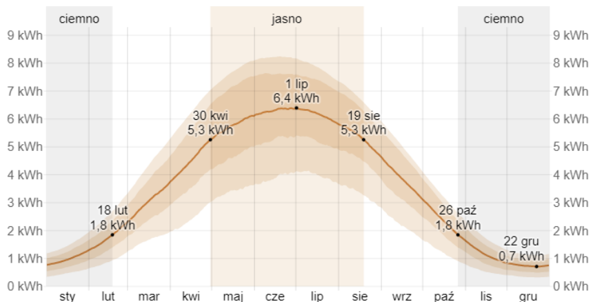
Wykres 6. Średnie dobowe padające promieniowanie krótkofalowe słoneczne w gminie Łaziska na przestrzeni roku
