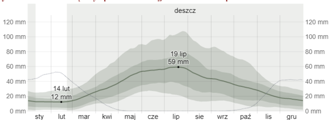
Wykres 4. Średni miesięczny opad deszczu w gminie Łaziska na przestrzeni roku
