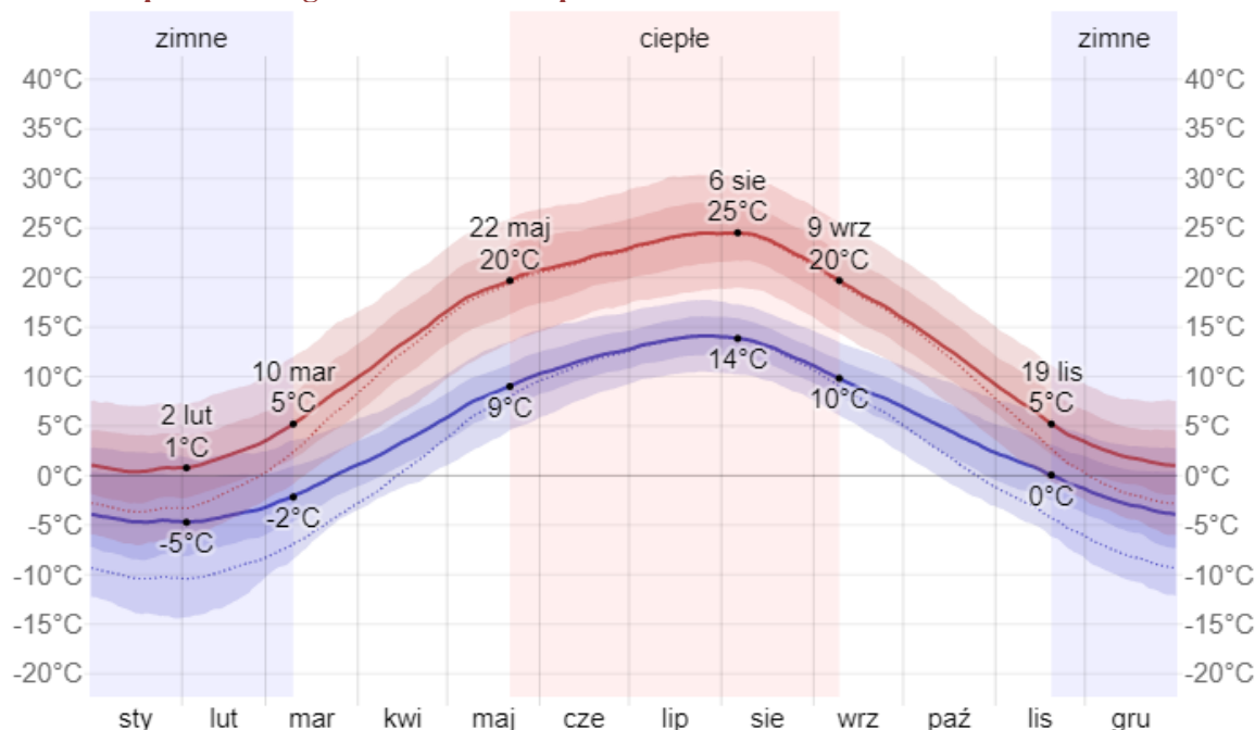
Wykres 2. Temperatura w gminie Łaziska na przestrzeni roku
